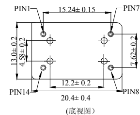
(底视图)
