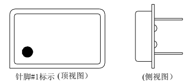
引脚#1标示 (顶视图)
