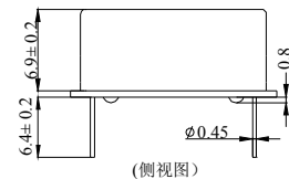
(侧视图)
